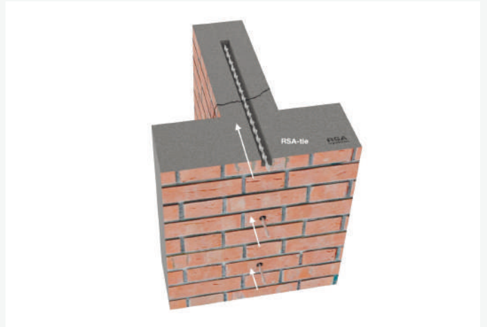
Рис. 8 Соединение внешней и внутренней стены вар.2
