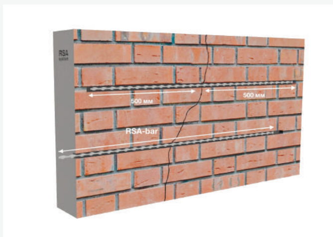
Рис. 1 Ремонт вертикальной трещины
