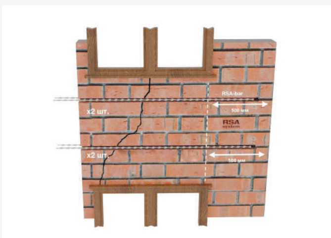
Рис. 5 Ремонт надоконной перемычки
