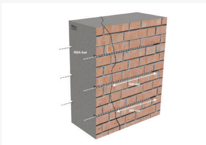
Рис. 4 Ремонт сквозной трещины
