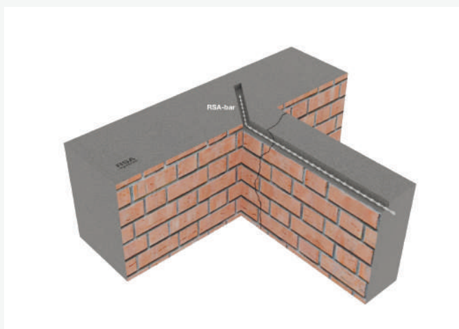
Рис. 3 Соединение внешней и внутренней стены
