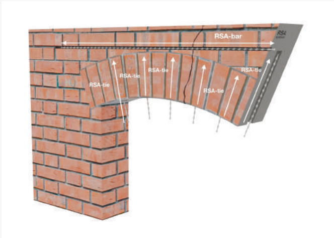
Рис. 7 Укрепление лучковой перемычки
