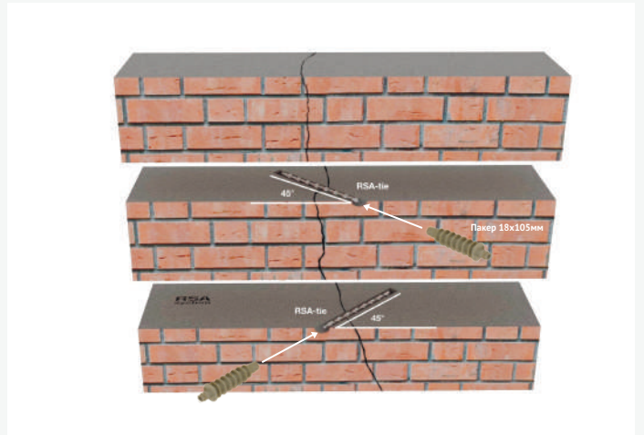
Рис. 10 Ремонт трещин «крестом» с одновременным инъецированием
