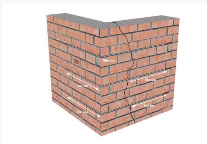
Рис. 2 Ремонт трещины на углу
